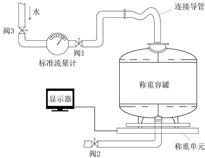
图1 称重容罐校准示意图
